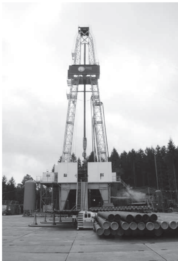
Urządzenie wiertnicze F400 w Równem.
