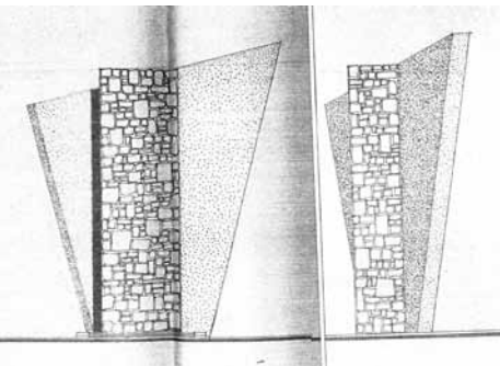
Widok projektu pomnika od strony bramy cmentarnej (z lewa) oraz widok boczny
