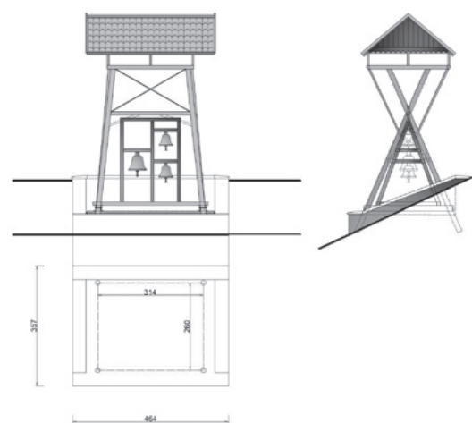
Dzwonnica na Pustelni Św. Jana z Dukli. Fragment projektu technicznego autor. dr inż. Marka Gransickiego
