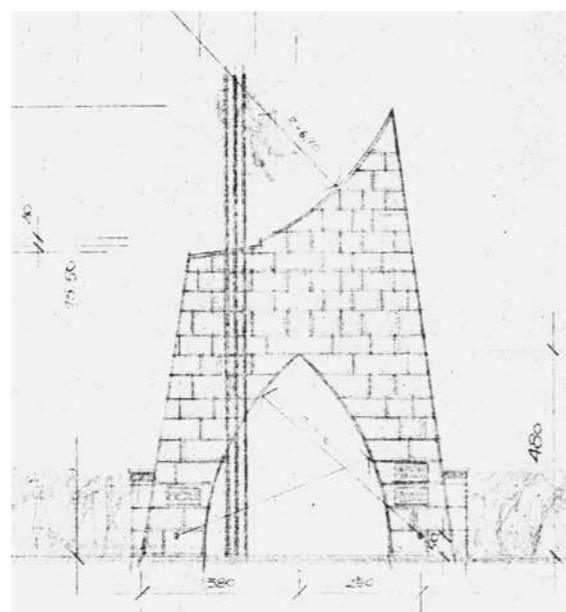
Fragment projektu bramy cmentarza wojennego w Dukli autorstwa architekta mgr inż. Stanisława Paprowicza
