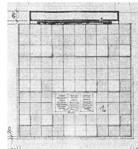
Druga wersja projektu płyty pomnika z murem i płaskorzeźbą na cmentarzu wojennym w Dukli autorstwa architekta Stanisława Pąprawicza
