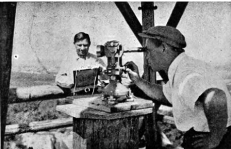
Pomiary katowe metodą Schreibera wykonywane w 1935 roku teodolitem WILDA ze stolika obserwacyjnego wieży triangulacyjnej Czartowska Skala pod Lwowem (wysokość 47,6 m, wysokość kozła 35,0 m) sieci I rzędu
