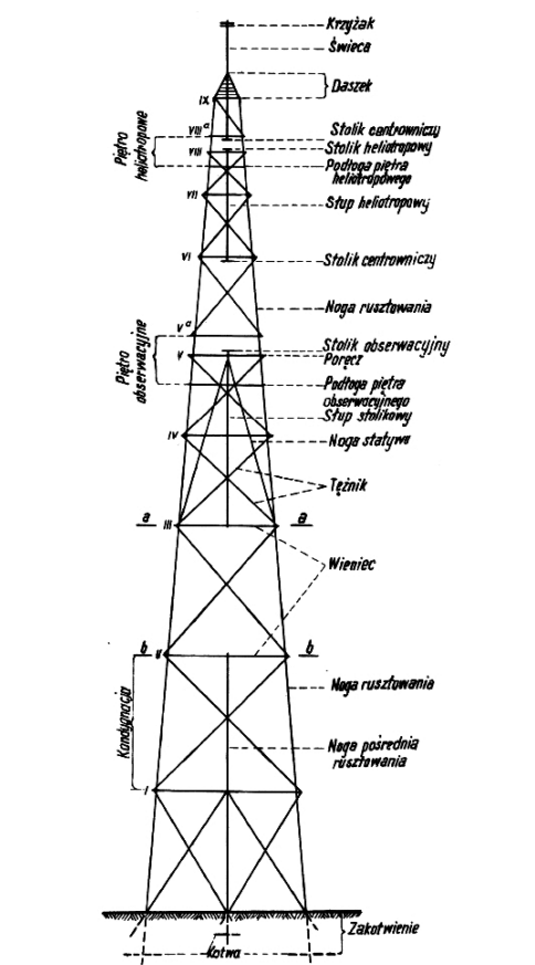
Wieża triangulacyjna drewniana stała 4/4, wysokość około 50 metrów – tego typu budowla została wzniesiona w latach trzydziestych XX wieku na górze Cergowa
