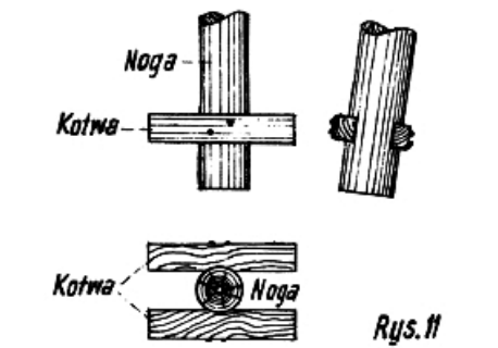
Nogi wieży triangulacyjnej zabezpieczone kotwami
