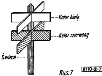
Szczyt świecy z krzyżakiem wieży triangulacyjnej
